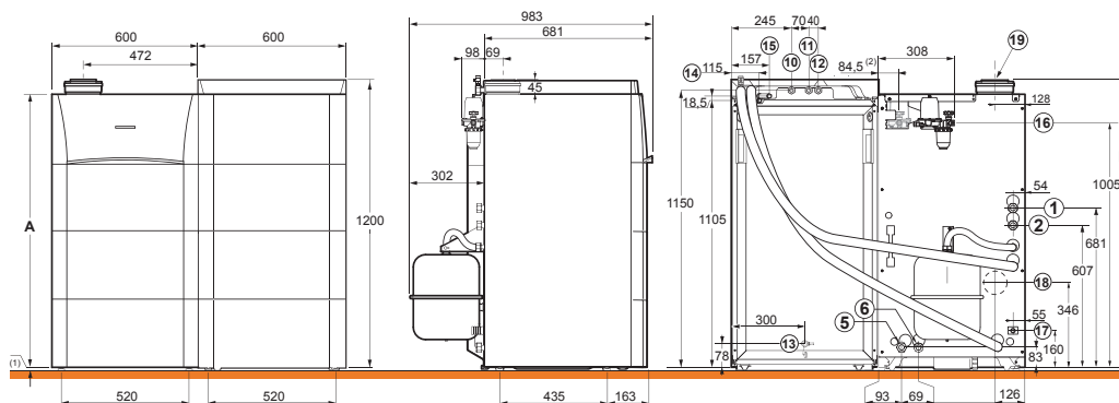
Bollitore 220 SHL
